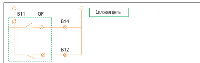
Схема подключения
