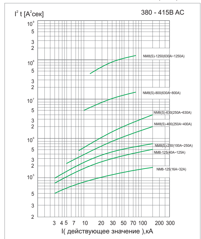
A^2сек характеристика
