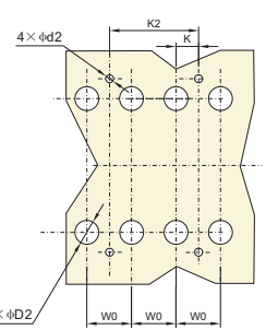
4 - х полюсные
